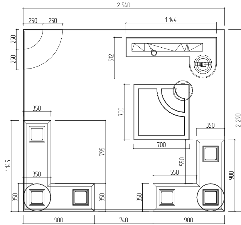
Вид сверху
