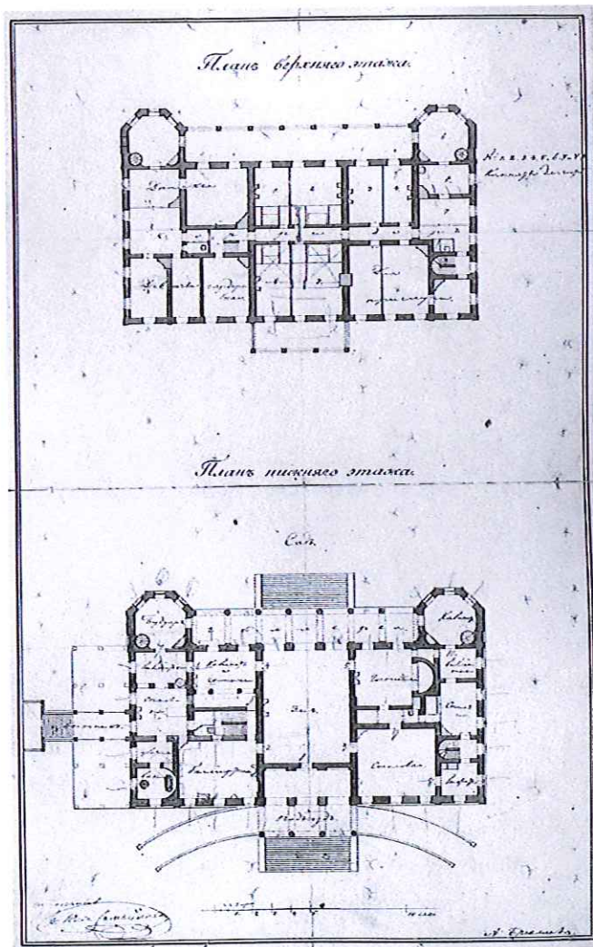
Рис. 5, 6 Проект усадебного дома графини Ю.П. Самойловой, 1830 г., арх. А.П. Брюллов
