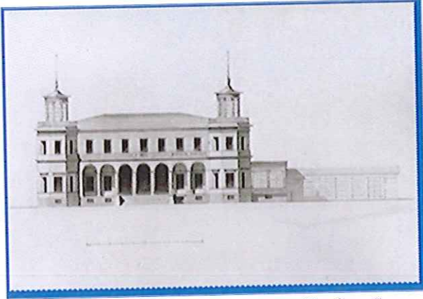
Рис. 7 Эскиз проекта здания в Графской Славянке 1830 г., арх. А.П. Брюллов
