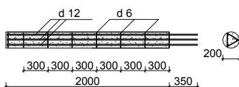
Каркас №4 - свая d 200
